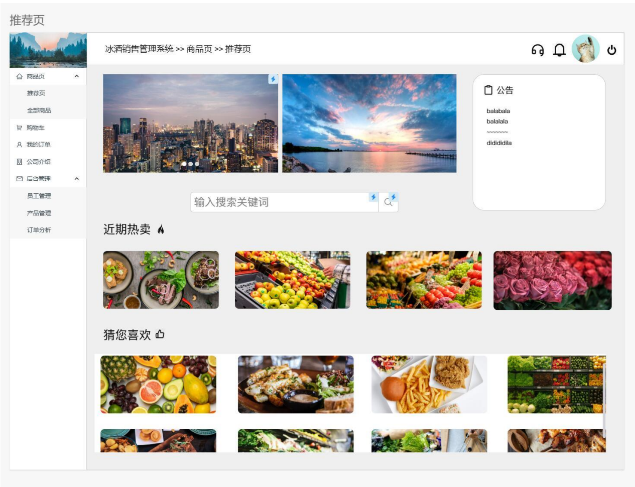
图 5.3：推荐页面
