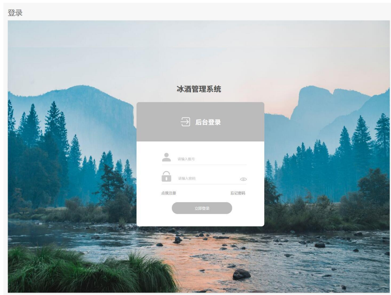
图 5.1：登录页面
