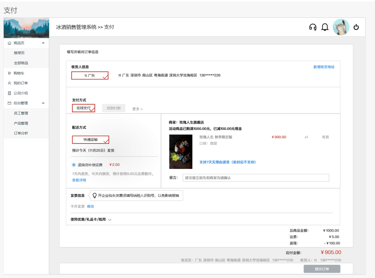
图 5.6：支付页面
