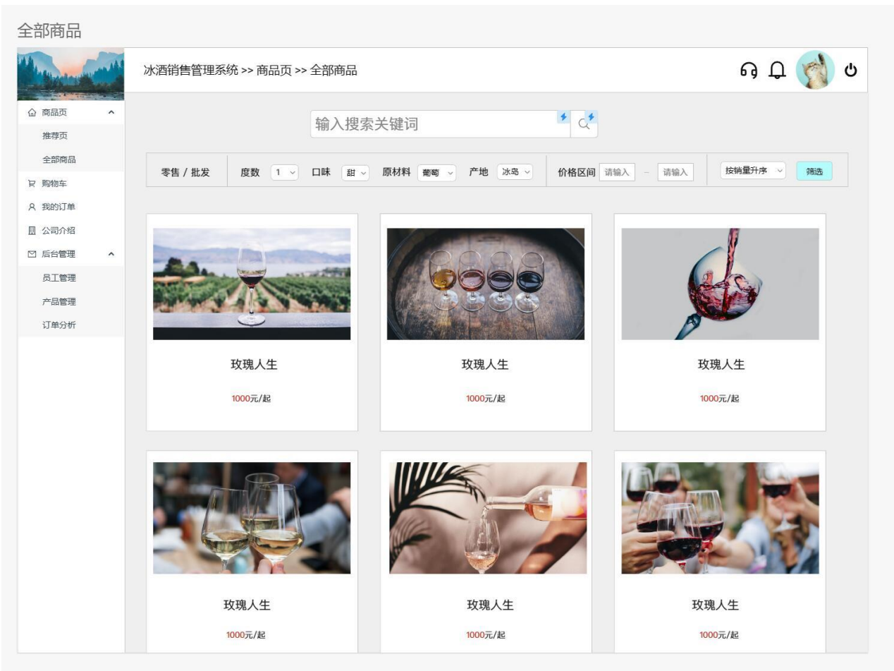
图 5.4：商品页面
