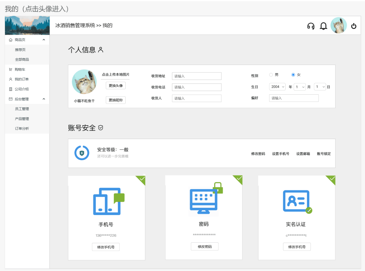
图 5.9：我的页面
