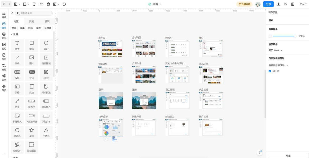
图 5.17：总览
