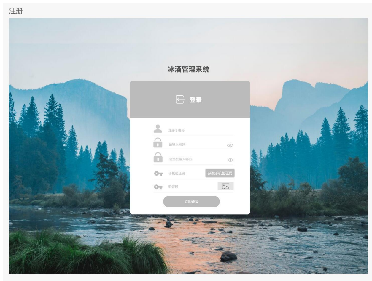
图 5.2：注册页面
